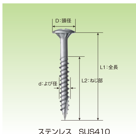
■ステンレスSUS410 ニュー雨樋ビス
