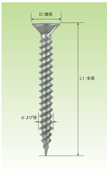
■軽天タッピング フレキ
