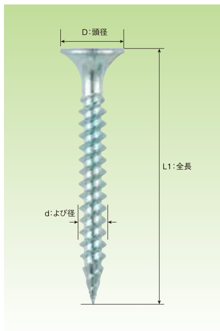
■軽天タッピング ラッパ
