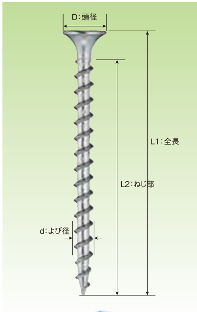
■ ステンレスSUS410 コーススレッド ラッパ 小箱
