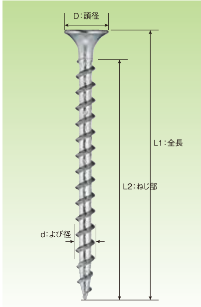
■ ニューステンレス コーススレッド(SUS410) ラッパ 小箱
